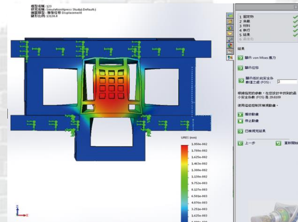
机台本体应力分析。
