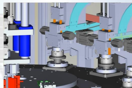
插入磁鐵
